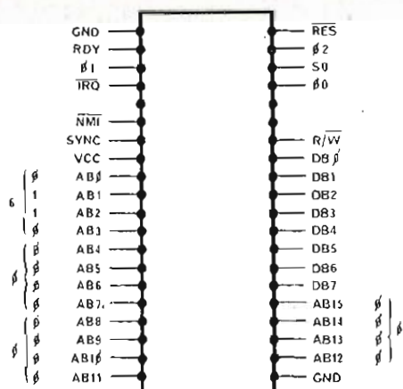
ZOCCOLATURA DEL MICROPROCESSORE 6502
